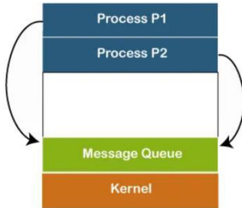
Передача данных
