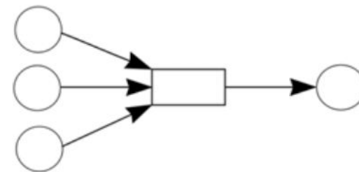
в) N — 1
