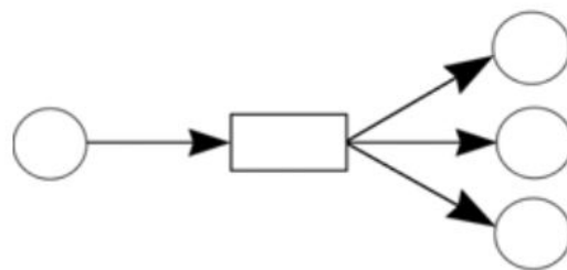
б) 1 — N
