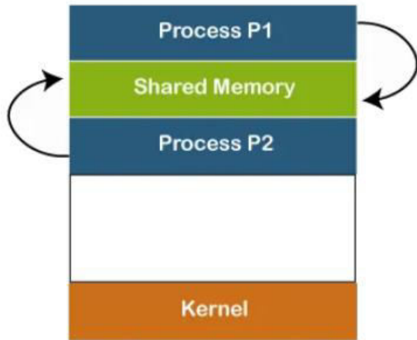
Разделяемая память
